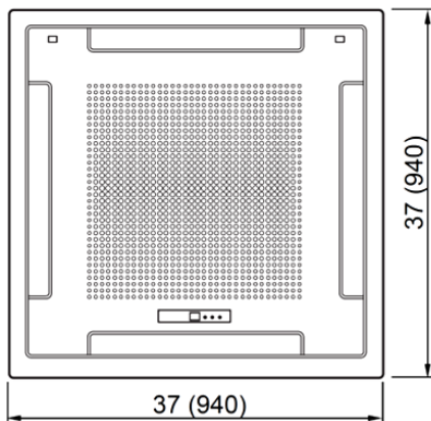
Bottom view (Panel)
