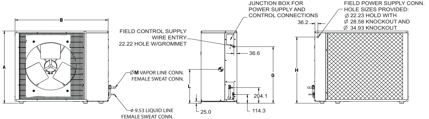
Fig. 5 — Dimensions
