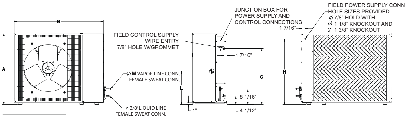
Fig. 3 — Dimensions
